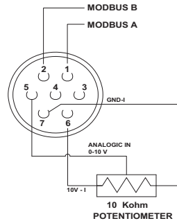
DETAIL VERBINDUNGEN
