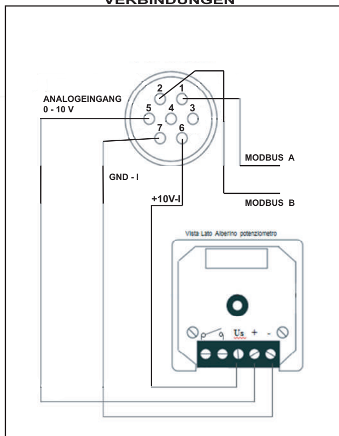
DETAIL VERBINDUNGEN
